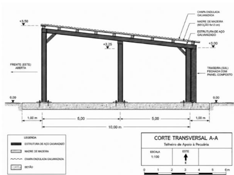
Figura 30: Corte transversal: estrutura de aço galvanizado, madres de madeira e cobertura inclinada para sul.
