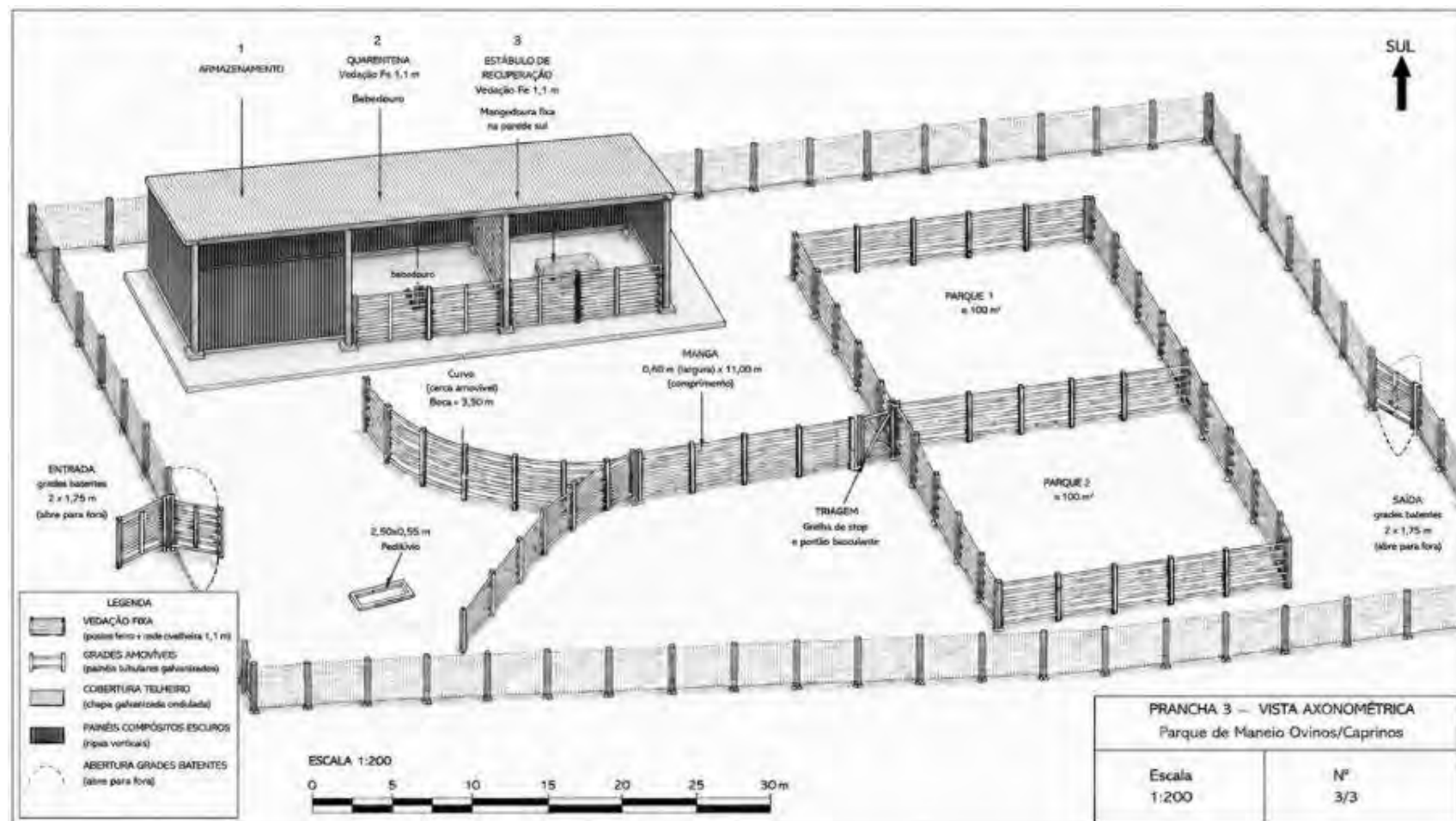
Figura 28: Vista axonométrica da solução funcional proposta.
