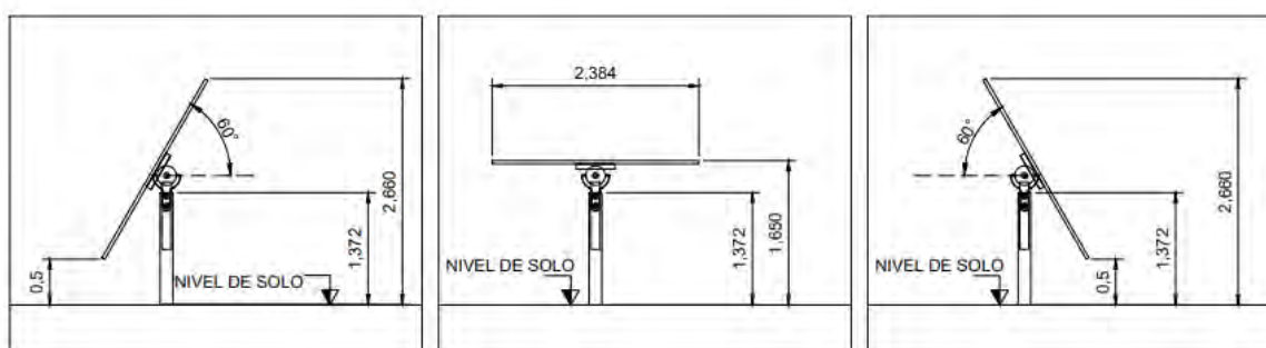
Figura 3: Sistema axial dos módulos fotovoltaicos da CSF (Fonte: EIA_CSF_Sophia).
