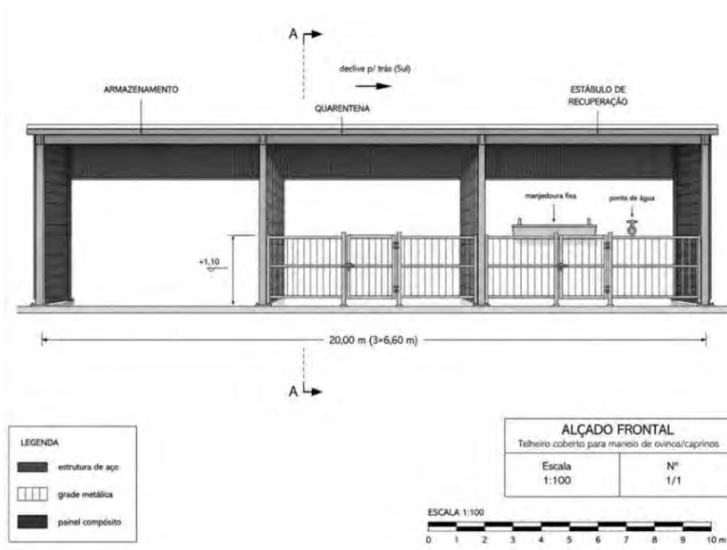
Figura 29: Alçado frontal do telheiro de apoio.
